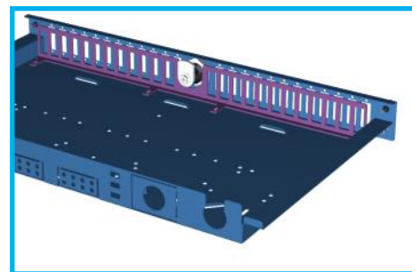
Opcjonalna płyta do bezśrubowego montażu adapterów światłowodowych
