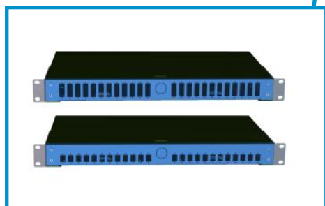
Zintegrowana płyta czołowa
