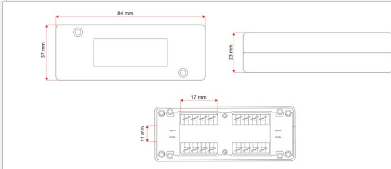
Rysunek techniczny
