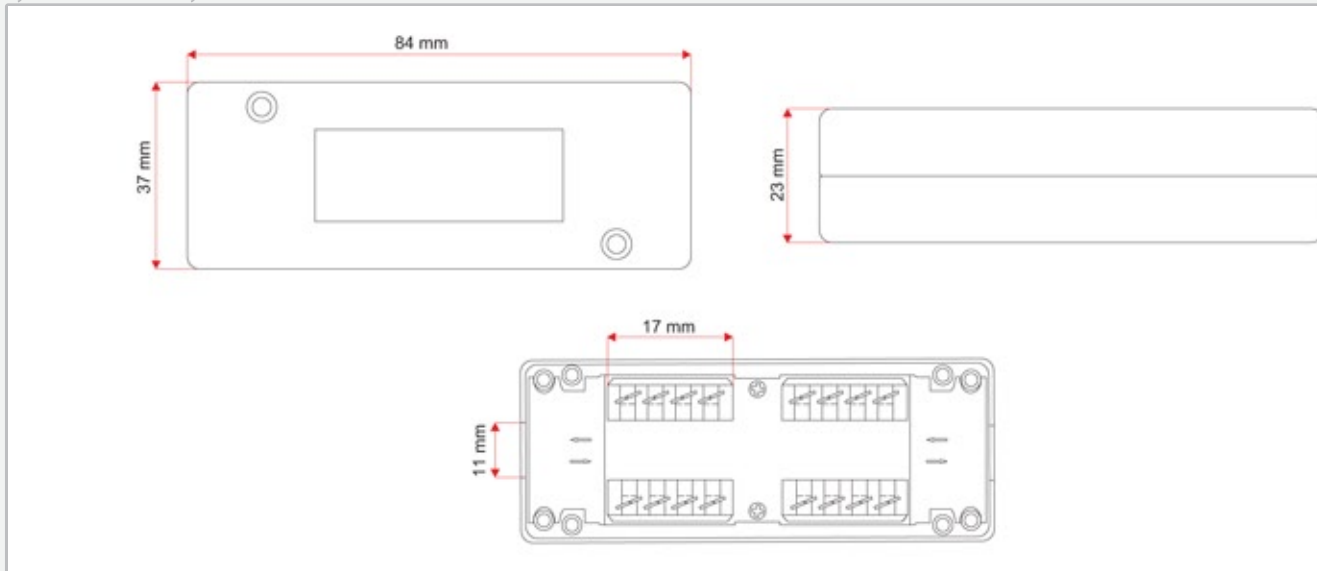
Rysunek techniczny
