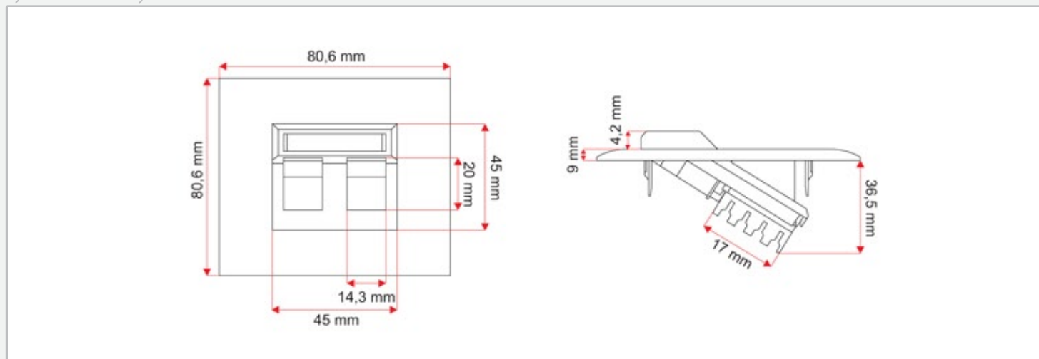
Rysunek techniczny
