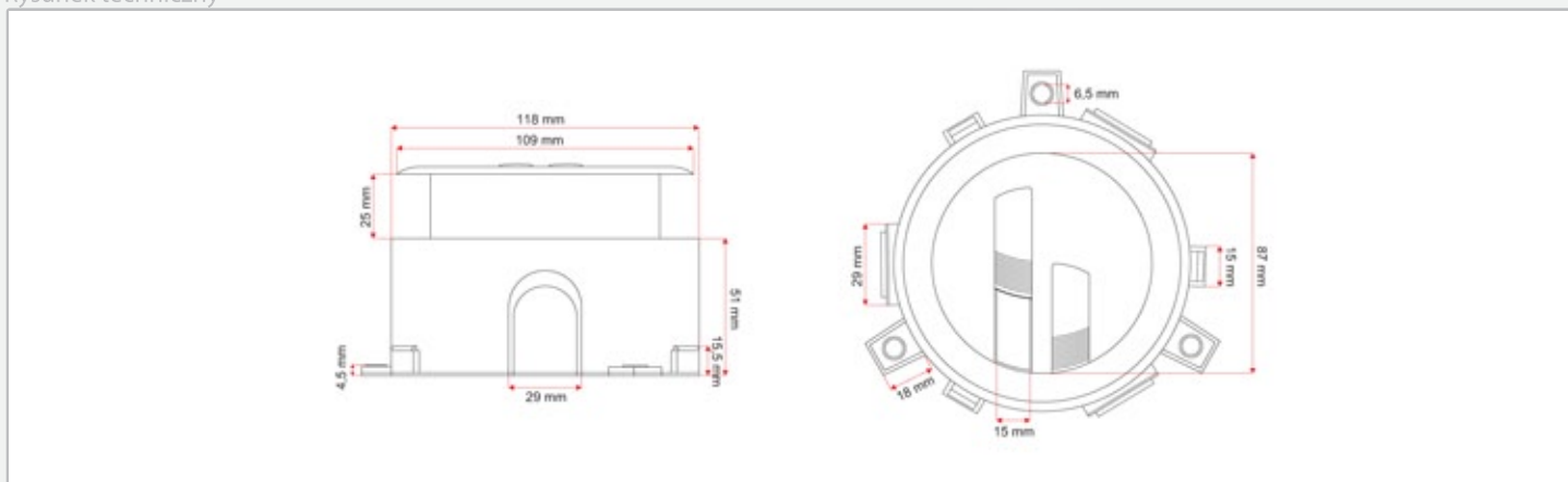
Rysunek techniczny
