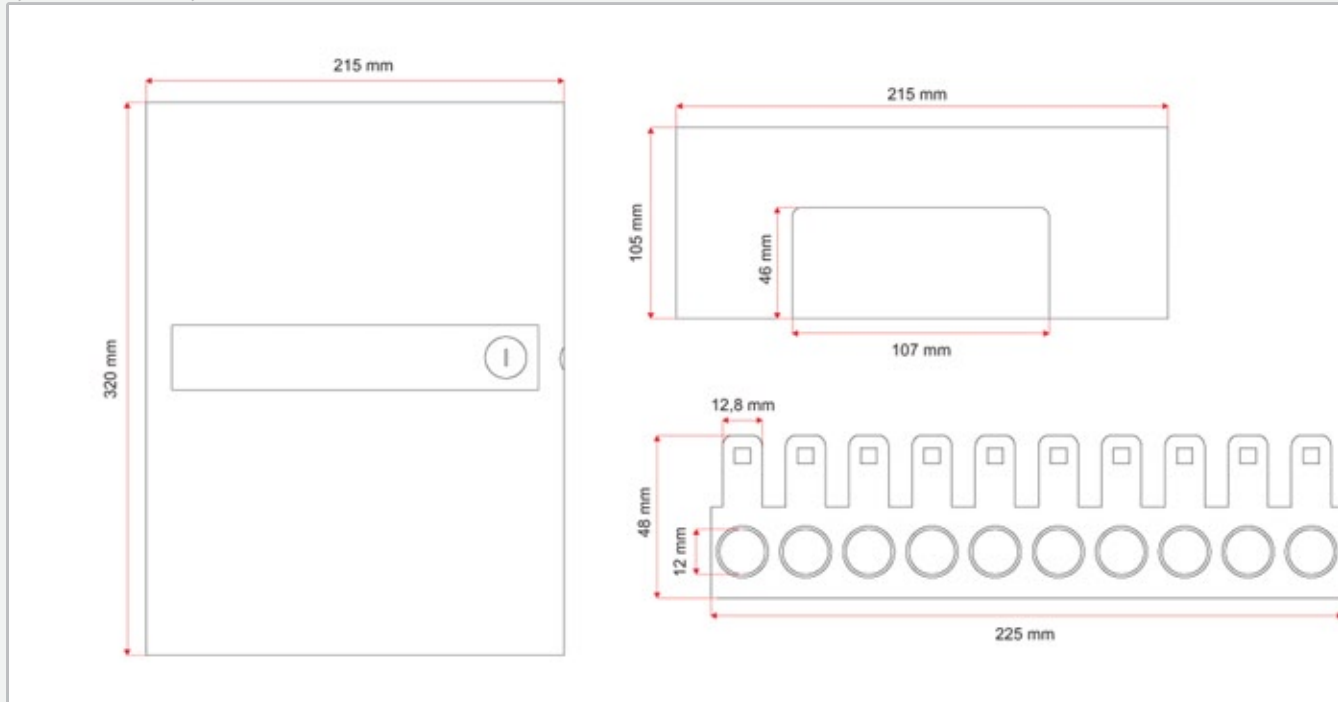
Rysunek techniczny
