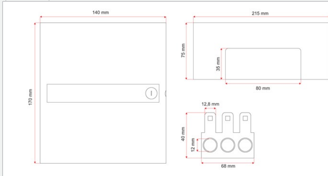
Rysunek techniczny
