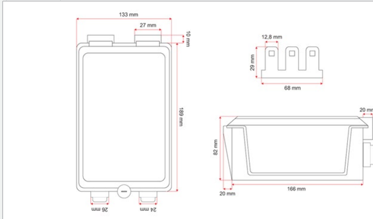
Rysunek techniczny
