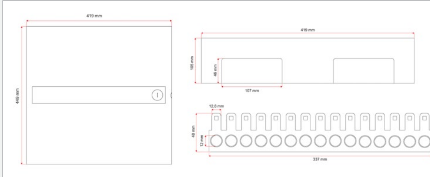
Rysunek techniczny
