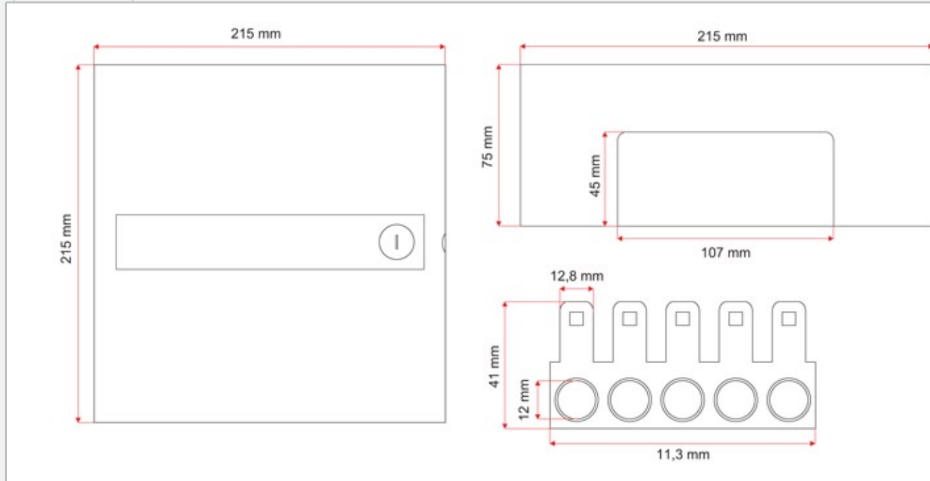
Rysunek techniczny
