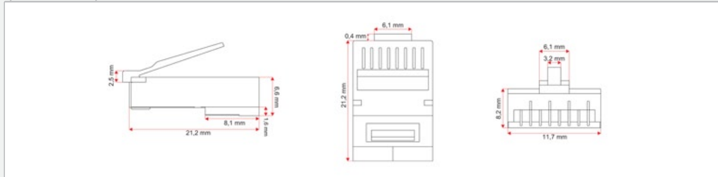
Rysunek techniczny
