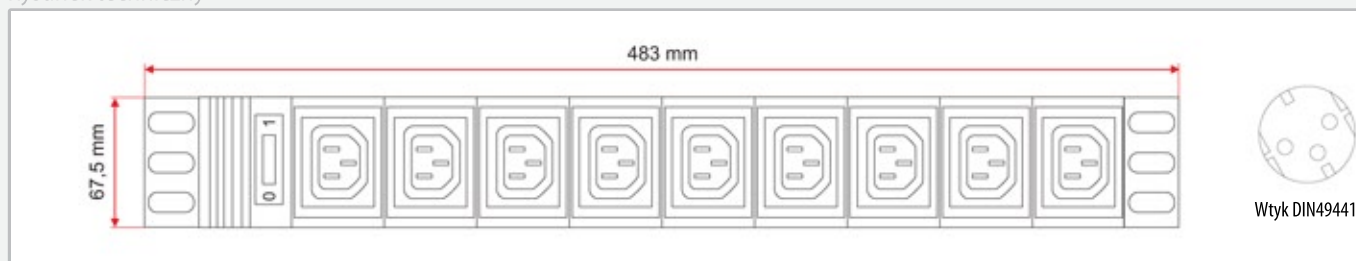
Rysunek techniczny
