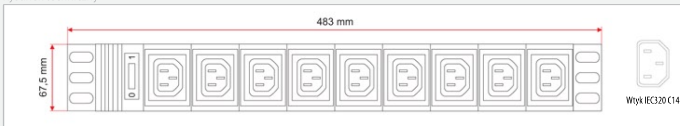
Rysunek techniczny
